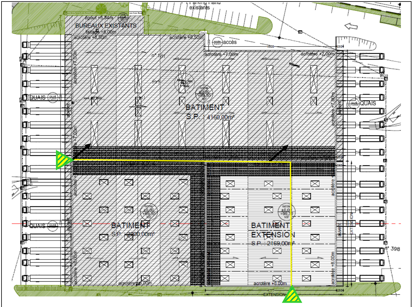
Plan n°3 : Implantation des paratonnerres, conducteurs de descente et prises de terre
