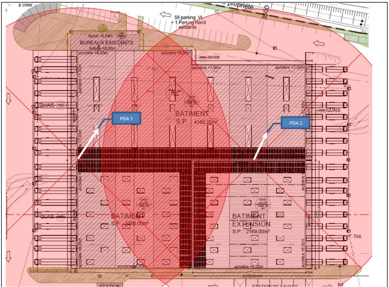
Plan n°2 : Rayon de protection des paratonnerres
