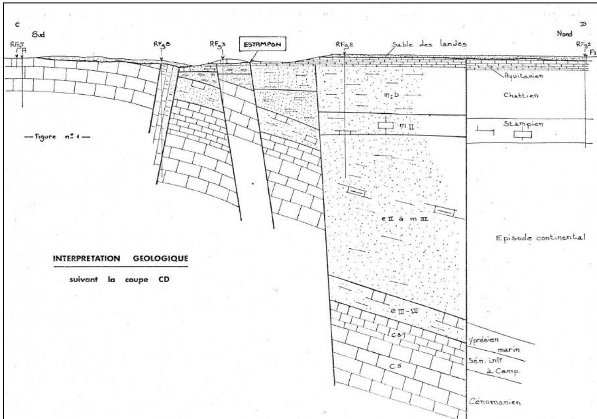
Figure 21 : Coupe géologique interprétative [Source : CETE]
