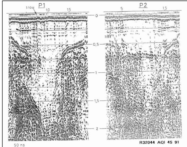
Figure 25 : Profils géoradar réalisés à l'aplomb d'un effondrement [Source : BRGM]
