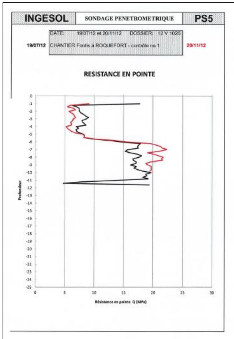
Figure 36 : Courbes des résistances en pointes réalisées en Juillet (en noir) et en Novembre 2012 (en rouge) du sondage PS5 [Source : INGESOL]
