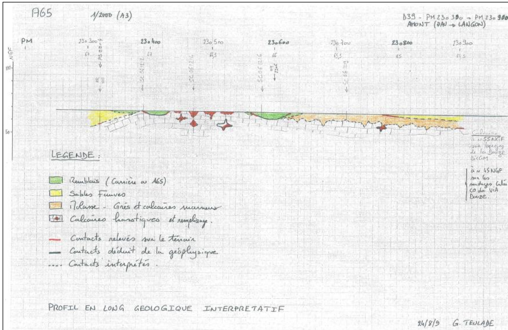
Figure 32 : Coupe géologique interprétative entre les PM 230 300 et 230 900 [Source : ARCADIS]
