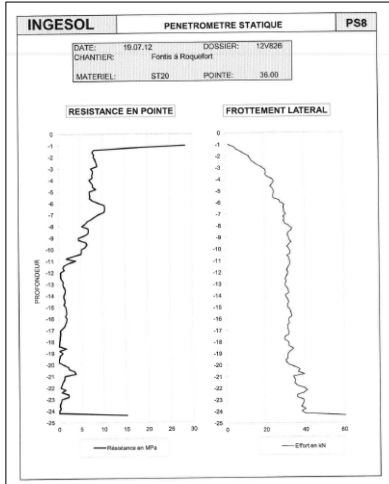
Figure 35 : Courbes de la résistance en pointe et du frottement du sondage PS1. A noter la présence d'une zone entièrement décomprimée entre 11 et 24 m [Source : INGESOL]
