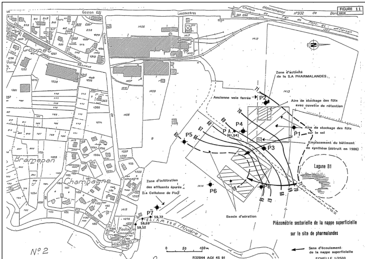
Figure 24 : Carte piézométrique du site PHARMALANDES [Source : BRGM]
