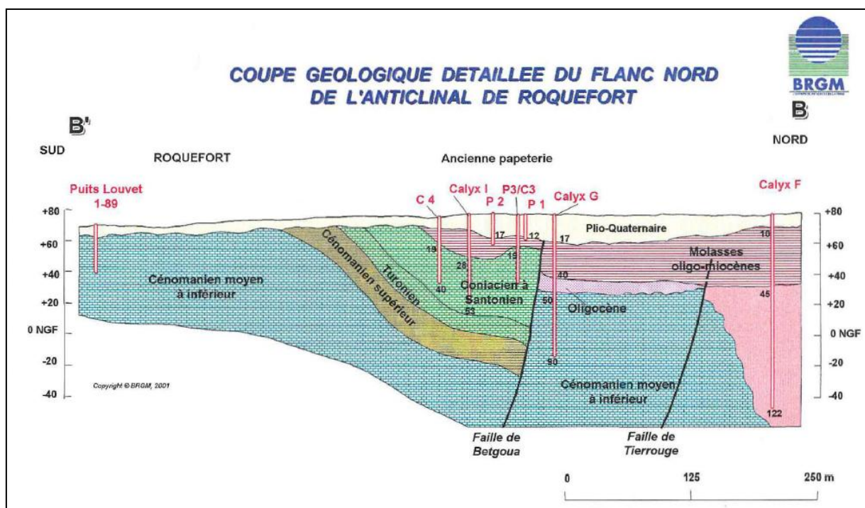
Figure 26 : Coupe géologique du flanc Nord de l'anticlinal de ROQUEFORT [Source : BRGM]
