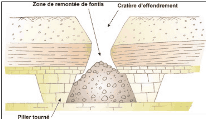
Figure 47 : Schéma [Source : BRGM] et photographie d'un fontis à ROQUEFORT [Source : IMS RN ]
