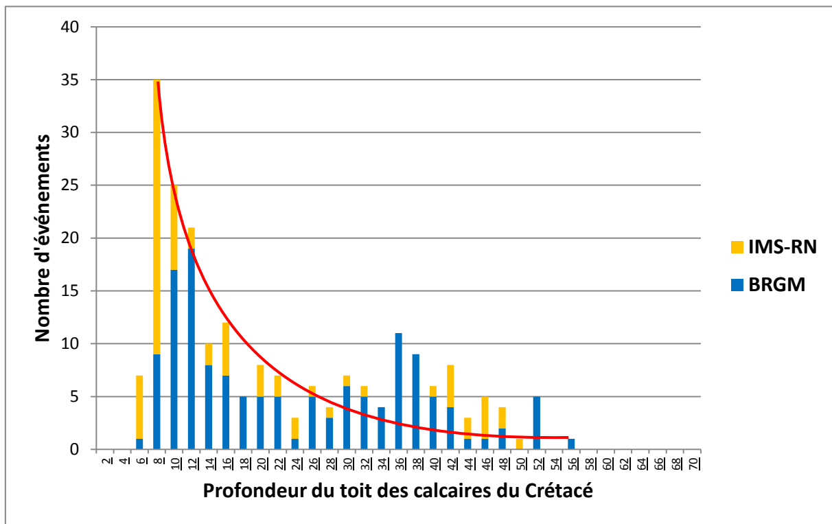
Figure 52 : Nombre de désordres recensés en fonction de la profondeur du toit des calcaires du Crétacé [Source : IMS RN ]
