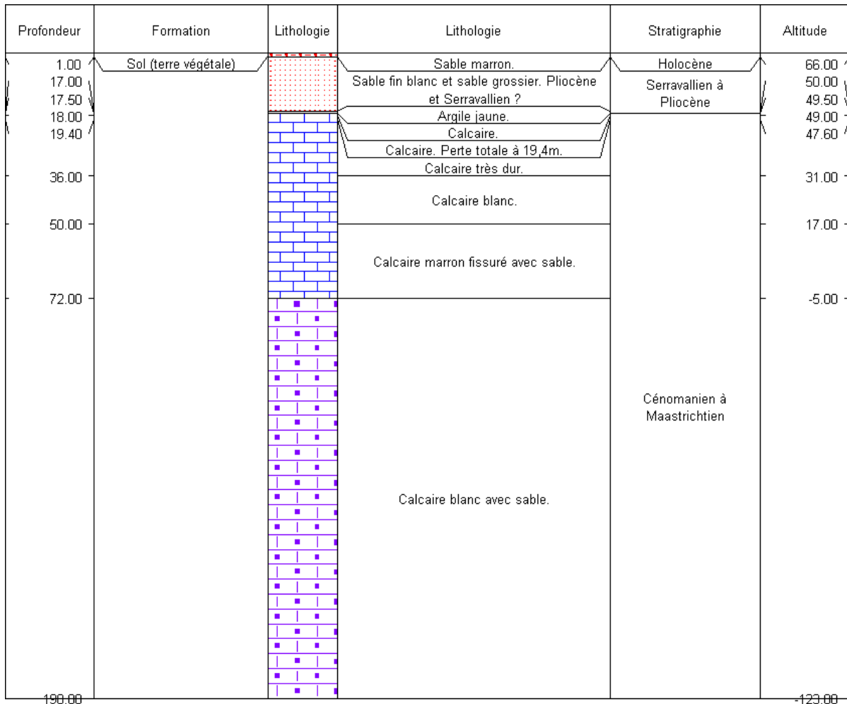
Figure 11 : Log géologique du forage n° 09261X0058/F1 [Source : BRGM]
