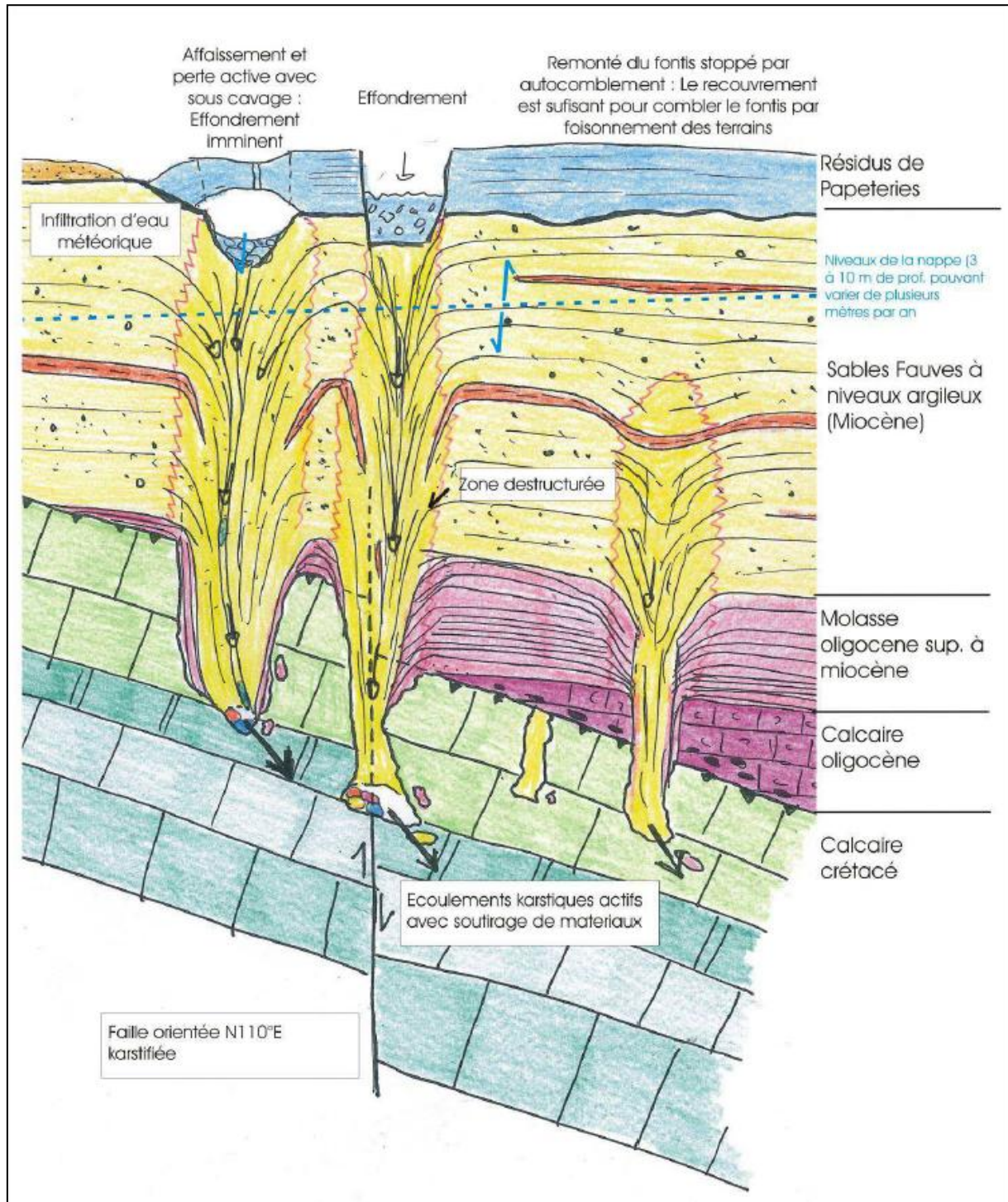
Figure 41 : Coupe schématique d'explication des désordres sur le site de SOCODAC [Source : BRGM]
