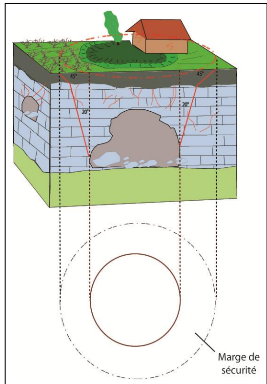
Figure 79 : Définition de la marge de sécurité : cas des effondrements de cavités souterraines [Source : IMS RN ]
