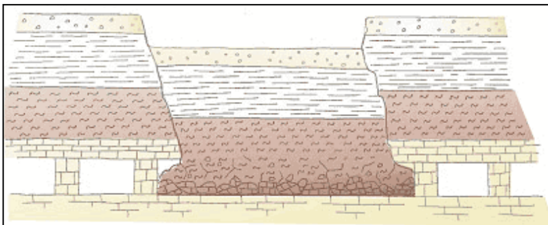
Figure 49 : Schéma [Source : BRGM] et photographie d'un effondrement généralisé à ST-EMILION (Gironde) [Source : CG 33]
