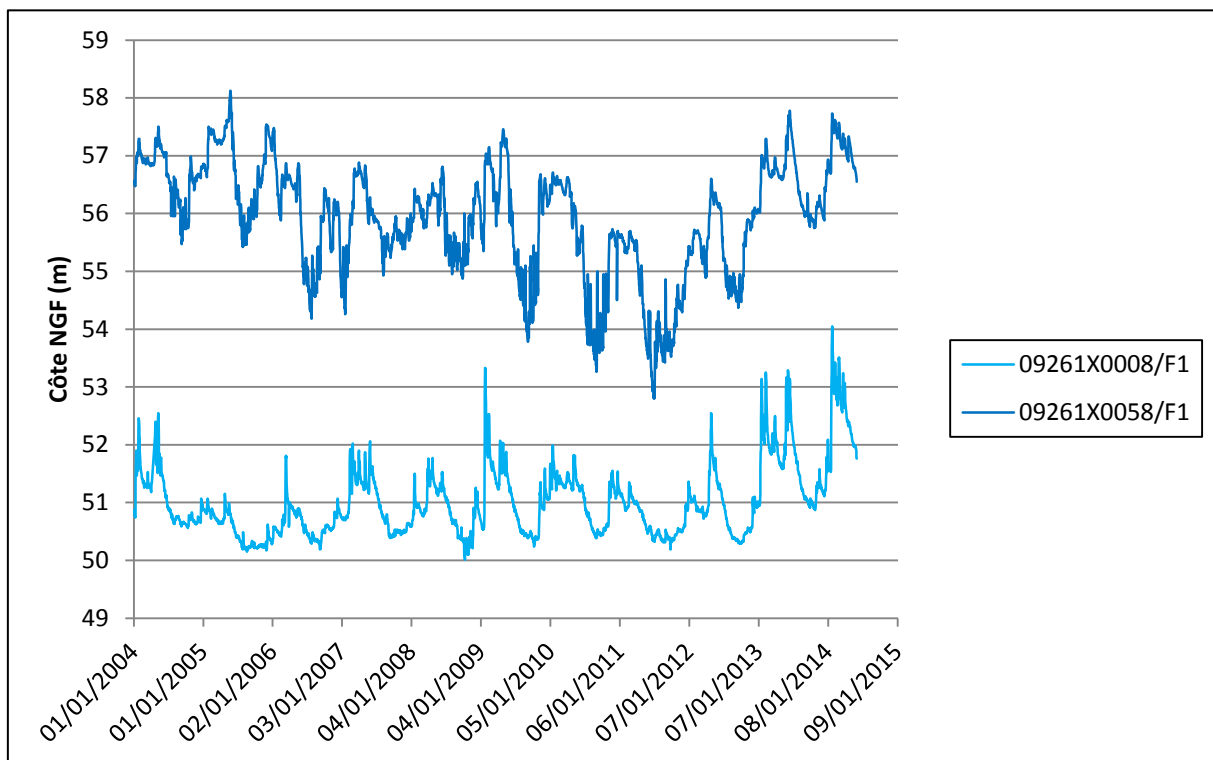
Figure 9 : Variation des niveaux piézométriques dans les forages n° 09261X0008/F1 et 09261X0058/F1, au cours de la période 2004-2014 [Source : ADES / IMS RN ]
