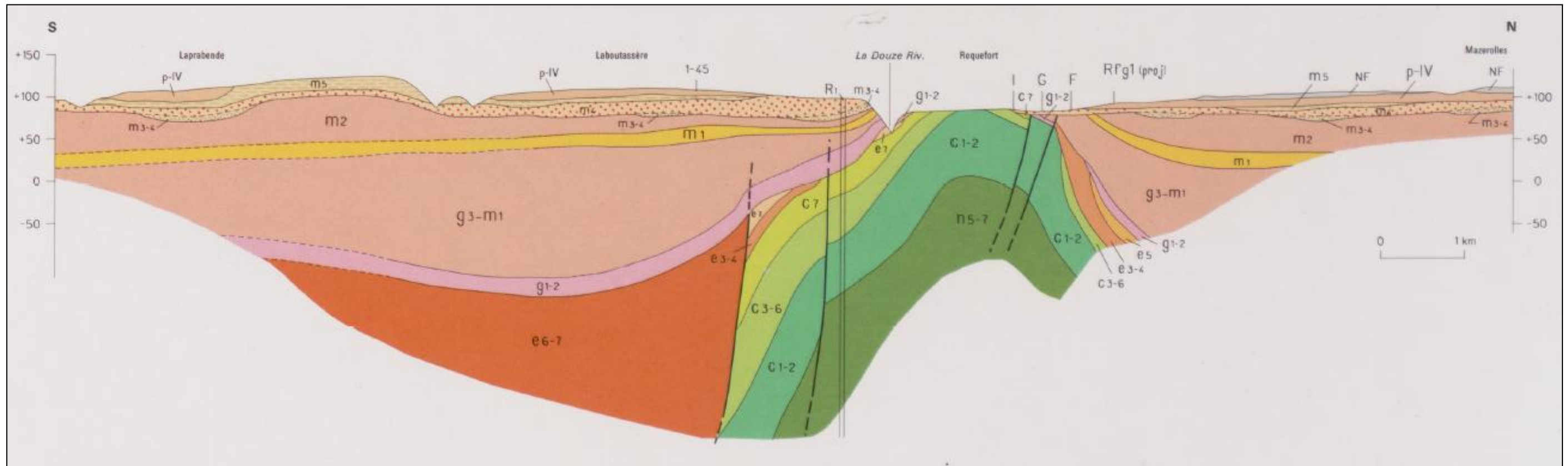
Figure 4 : Coupe géologique schématique traversant le dôme de ROQUEFORT [Source : BRGM]
