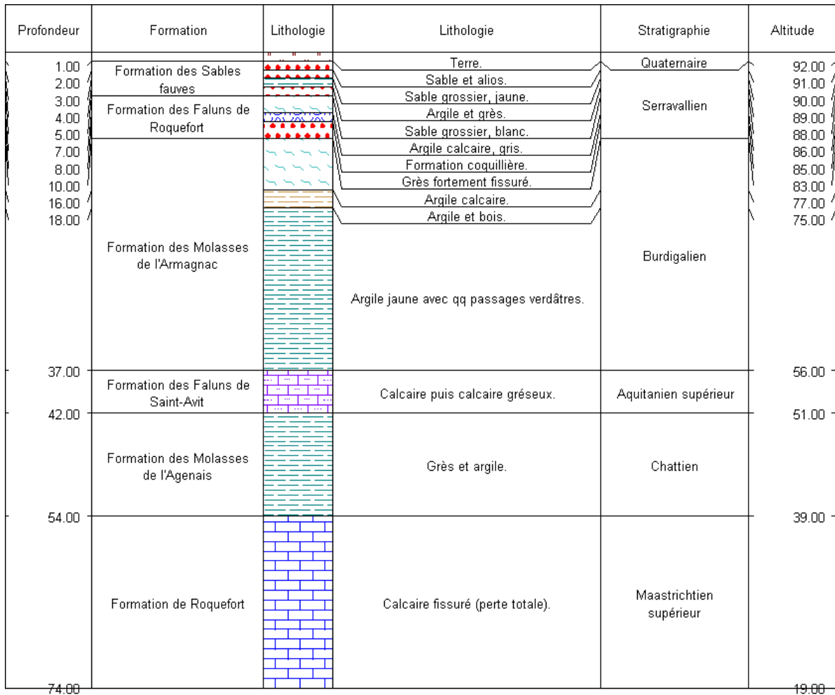
Figure 10 : Log géologique du forage n° 09261X0008/F1 [Source : BRGM]
