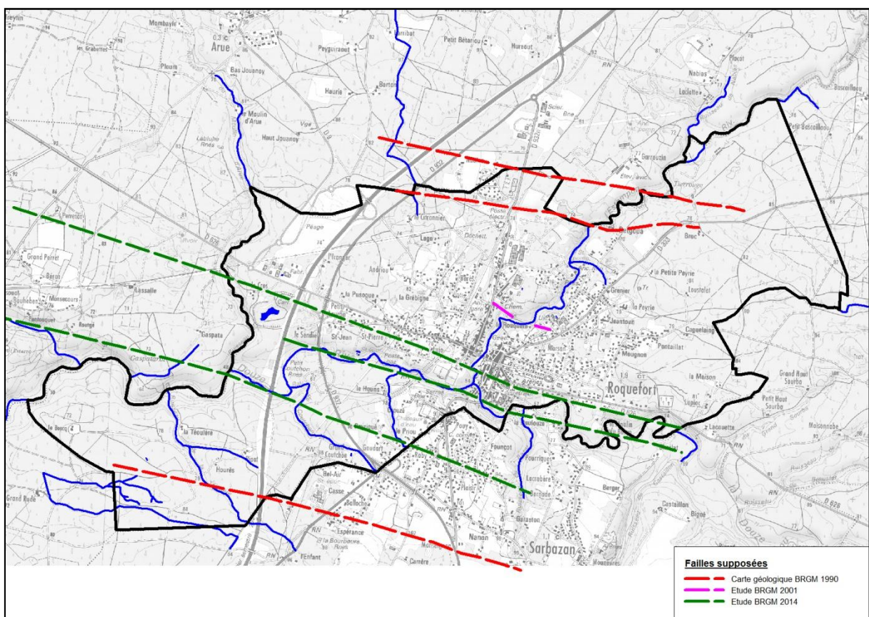
Figure 71 : Nouvelles failles ajoutés à la cartographie informative (en vert) [Source : BRGM / IMS RN ]
